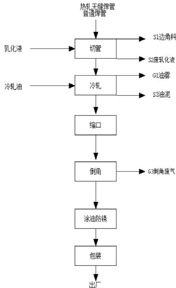
图 2-2 精密钢管生产工艺流程图
