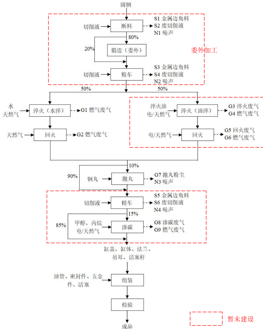
图 2-2 挖掘机油缸生产工艺流程图
