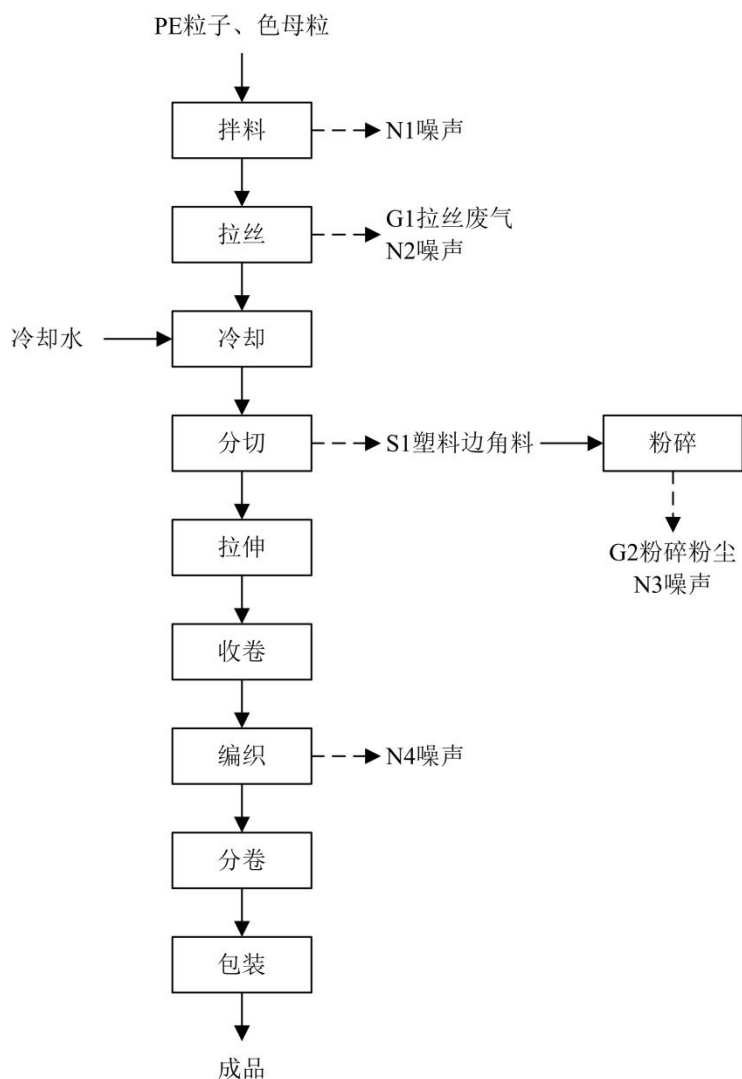
图 2-2 塑料遮阳网生产工艺流程图
