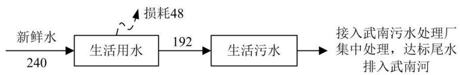
图 2-1 项目水平衡图 （单位：t/a）
